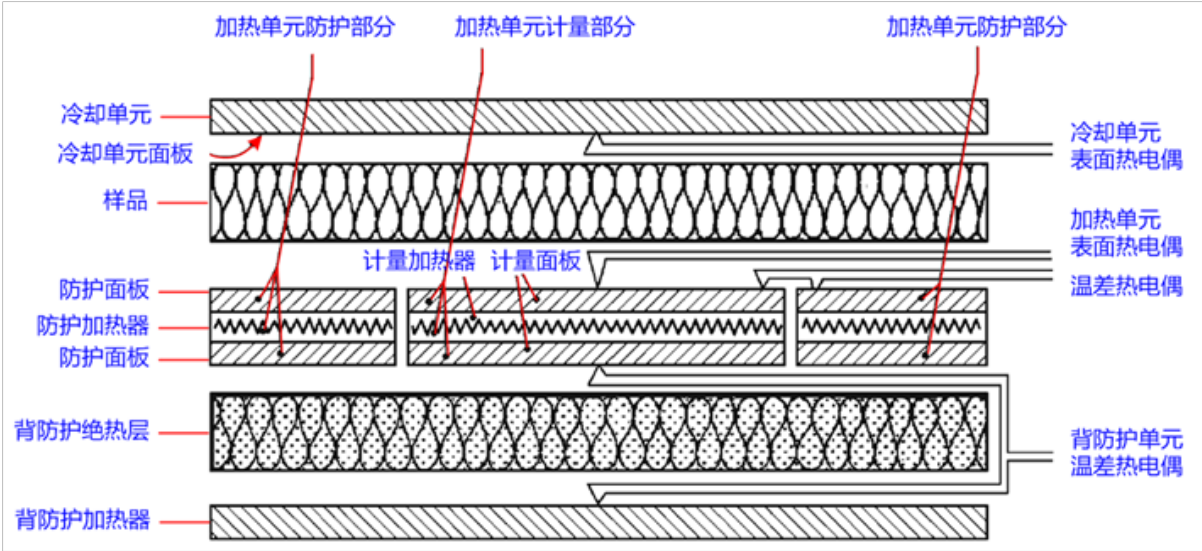
图 3-2 防护热板法单样品测试模型
